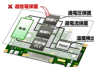
安全機構検証と改善提案(例)
