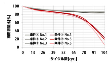
寿命評価設備と加速寿命試験結果(例)
